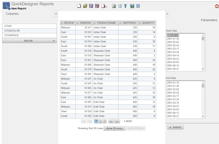
Parameters Pane
