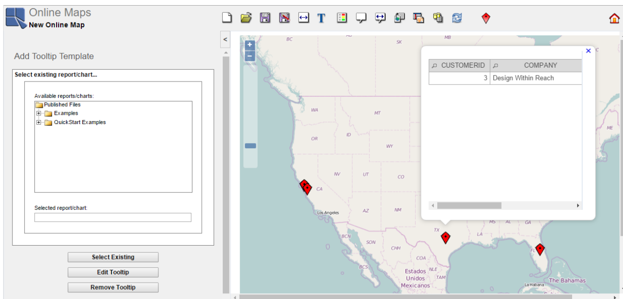
Adding Tooltip
