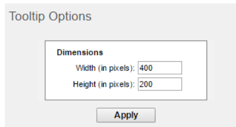
Tooltip Options
