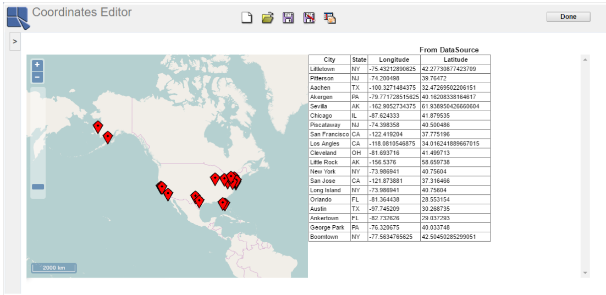
Coordinates Editor
