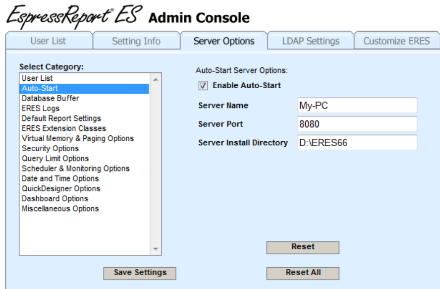
Auto-Start Options
